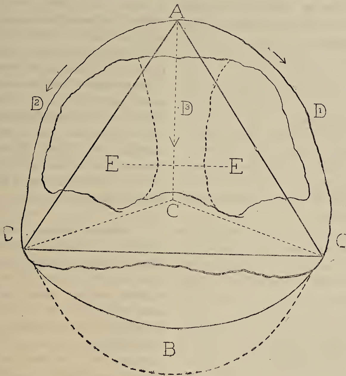
Fig. 2: A — African Pole (Polo Africano). B — Pacific Depression (Depressão do Pacifico). CC — Austral Bridge (Ponte Austral). D D D — Atlantic-Indian-Mediterranean Ring (Anel Atlantico-Indio-Mediterraneo). E E — Eria Bridge (Ponte Eria).
